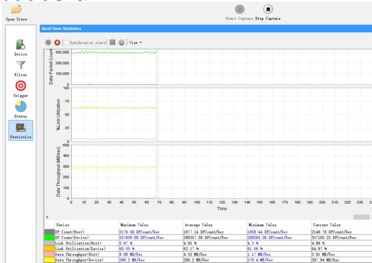
图 3-1 USB3 Agilent 分析仪测试传输速率
